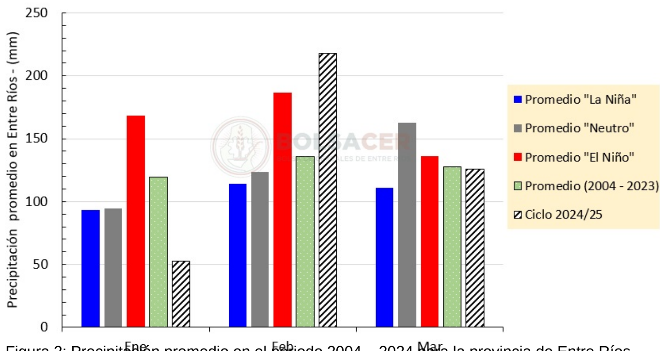
Figura 2: Precipitación promedio en el período 2004 – 2024 para la provincia de Entre Ríos entre los meses de enero a marzo, ciclo 2024/25 y los valores promedio históricos para eventos “El Niño” y “La Niña”.
