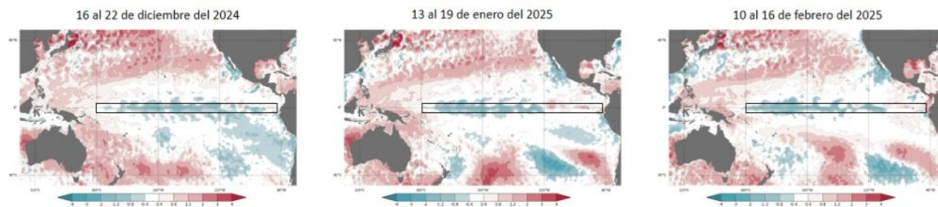
Figura 1: Diferencia con respecto a la observación de la temperatura de la superficie del mar en el Pacífico Ecuatorial. Fuente: www.cpc.ncep.noaa.gov
