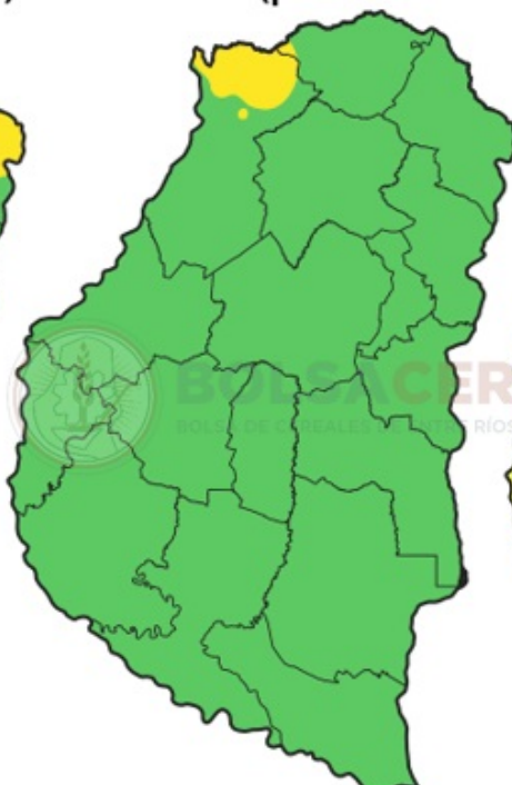
Precipitación promedio histórica (período 2004 - 2024)
