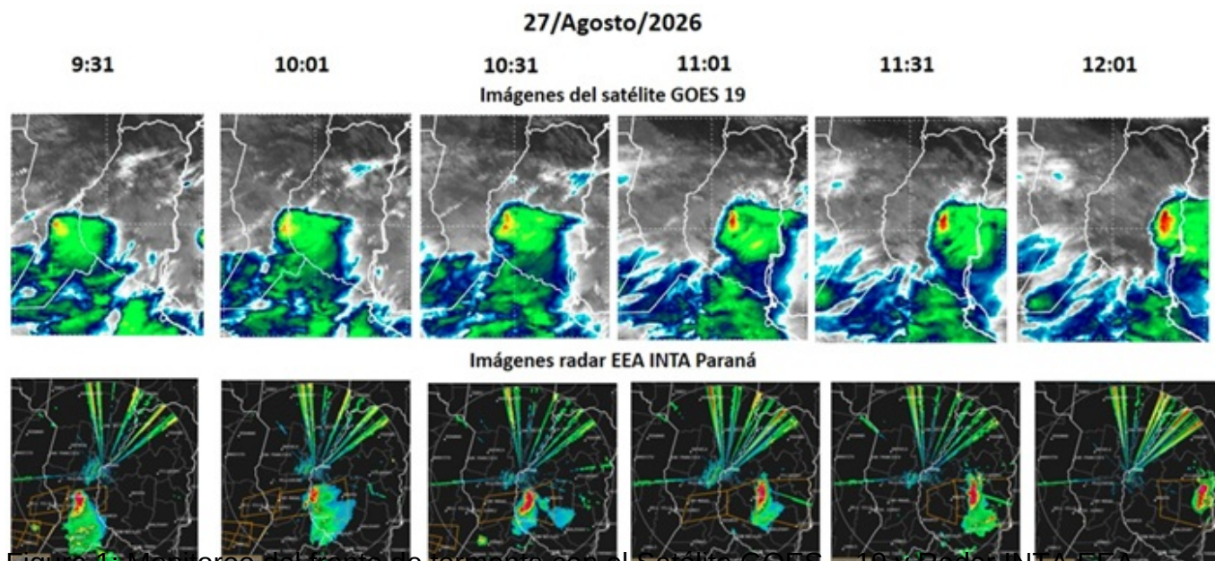
Figura 1: Monitoreo del frente de tormenta con el Satélite GOES 19 y Radar INTA EEA Paraná del jueves 27 de agosto.
